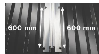
E Alternativ 2 – Med bärläkt. Bärläkt vid 600 mm c/c, skruva enligt bild och fortsätt likadant. Börja och avsluta med korta farmarskruv. Lång farmarskruv.
