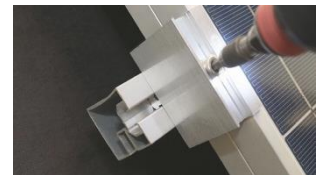
F. Skjut intill ändklämma mot solcellspanel och drag åt. Åtdragningsmoment 6–8 Nm
