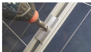
E. Skjut intill nästkommande solcellspanel och drag åt. Åtdragningsmoment 6–8 Nm
